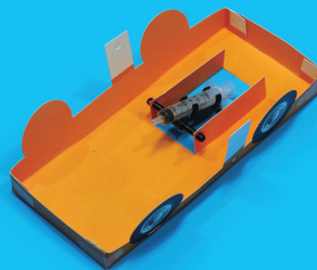
5 차체 아랫부분에 그림과 같이 샤프트를 끼우고 마개로 고정한 다음 차체의 날개부분의 홈을 샤프트에 끼워 차체가 벌어지지 않게 한다.
