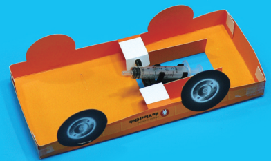
5 차체 아랫부분에 그림과 같이 샤프트를 끼우고 마개로 고정한 다음 차체의 날개부분의 홈을 샤프트에 끼워 차체가 벌어지지 않게 한다.
